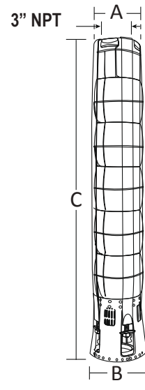
Acoplamiento NEMA 8"
